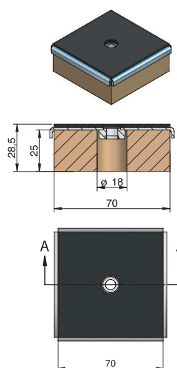
TSR con Kit de Nivelación
